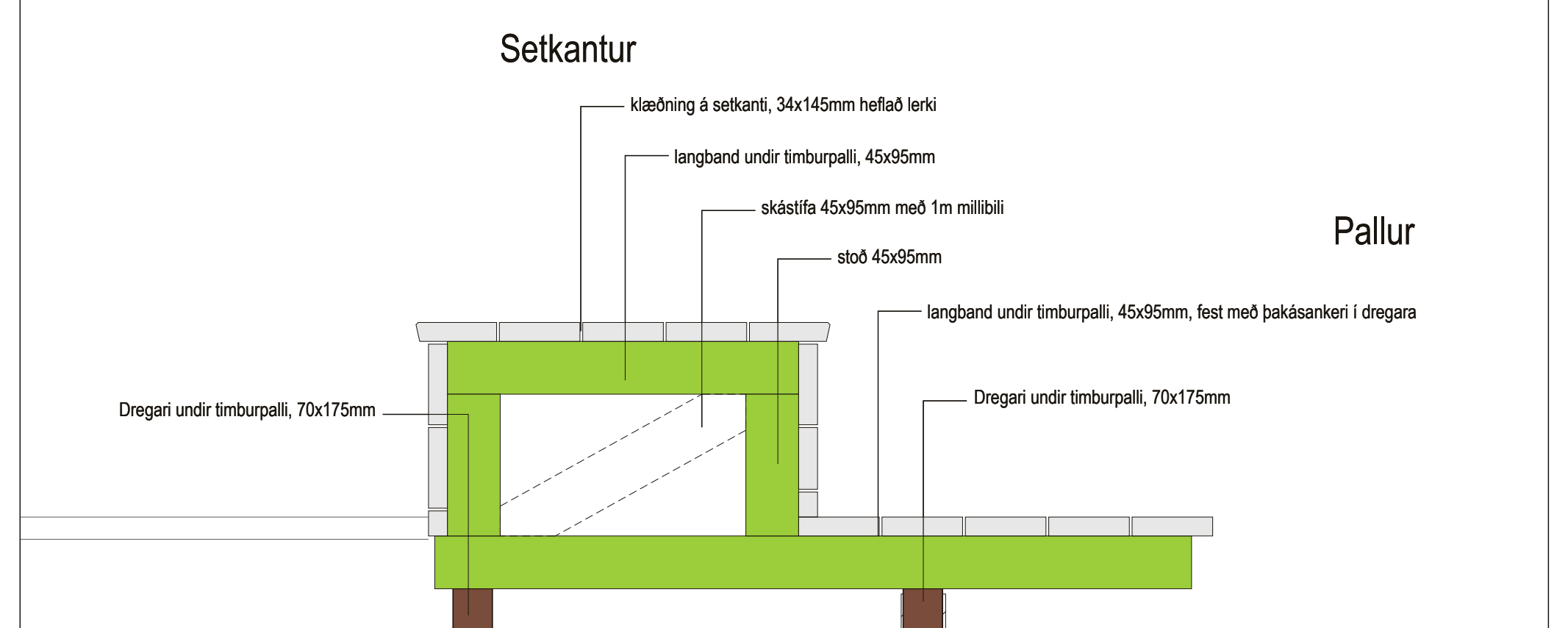
Setkantur - snið c-c' - Mkv. 1:10
