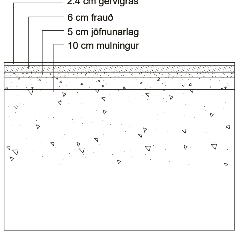
Sport-gervigras
