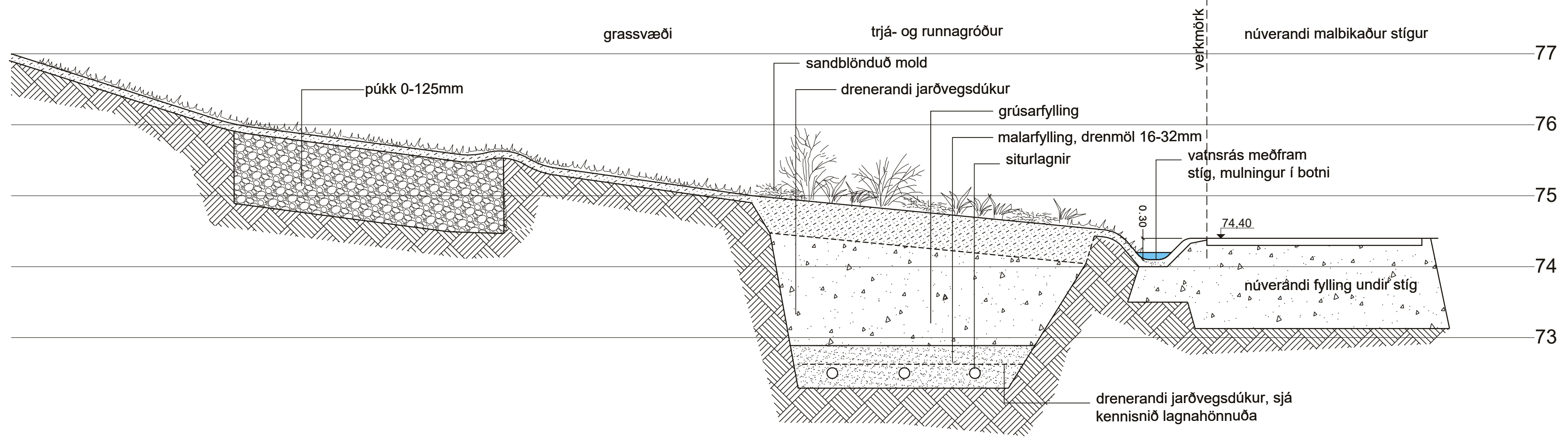
Snið F-F, mkv. 1:50
