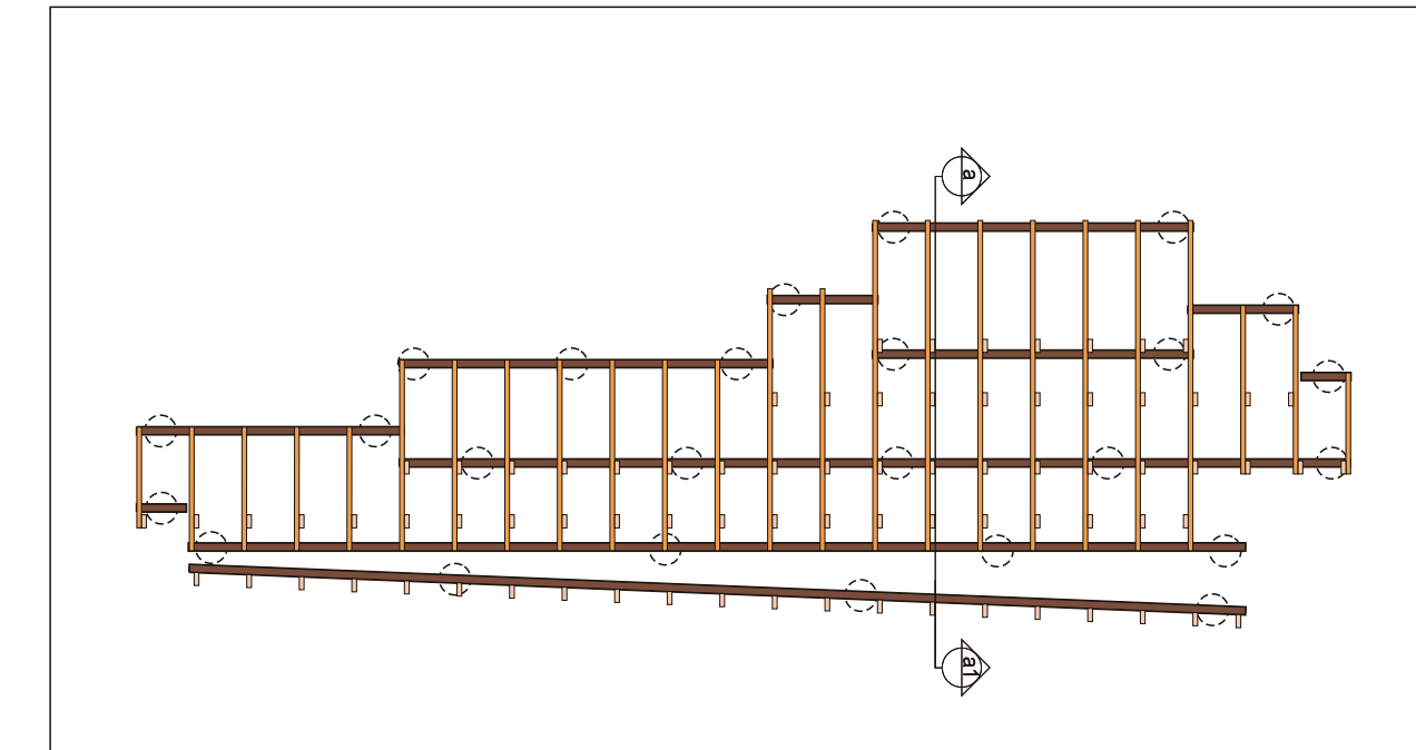
Uppistöður og dregarar - lárétir og ská dregarar
