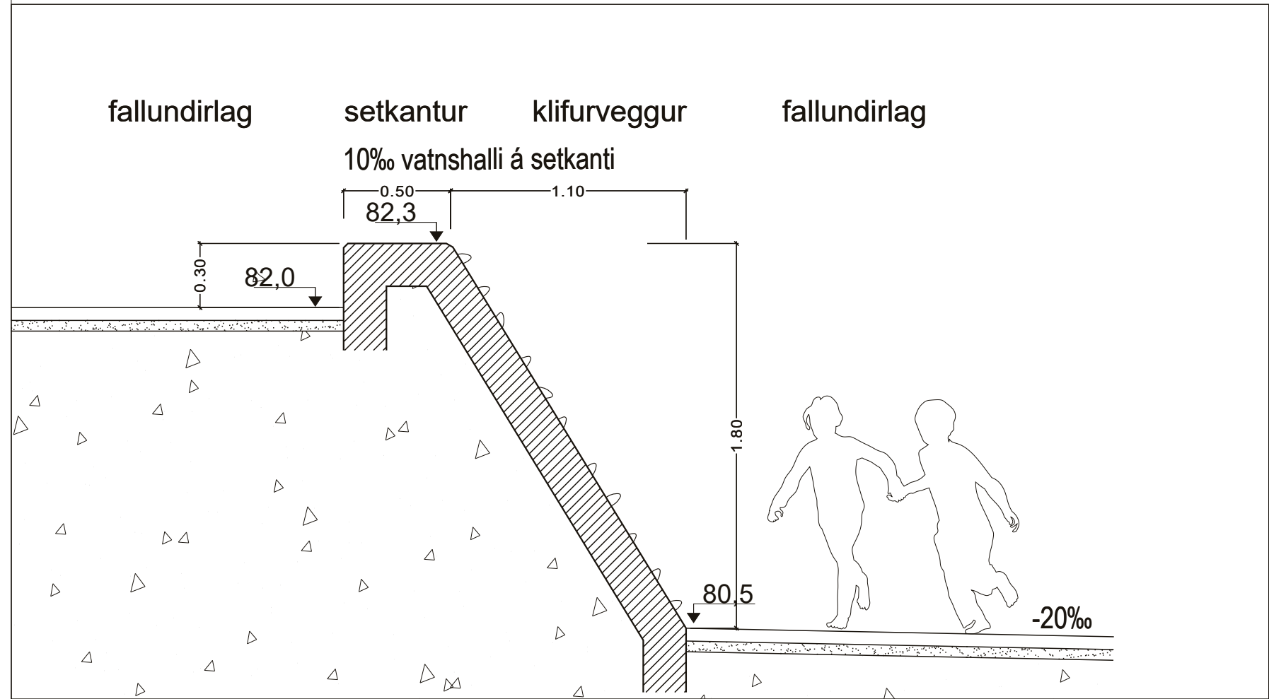
Veggur V-1 - snið a-a - Mkv. 1:25
