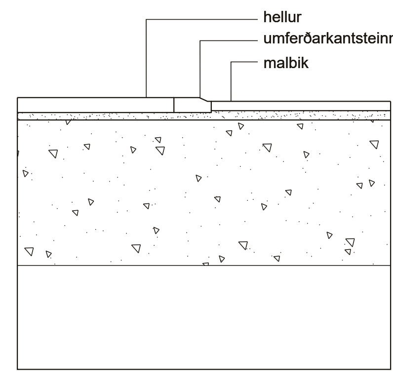
Umferðarkantsteinn
