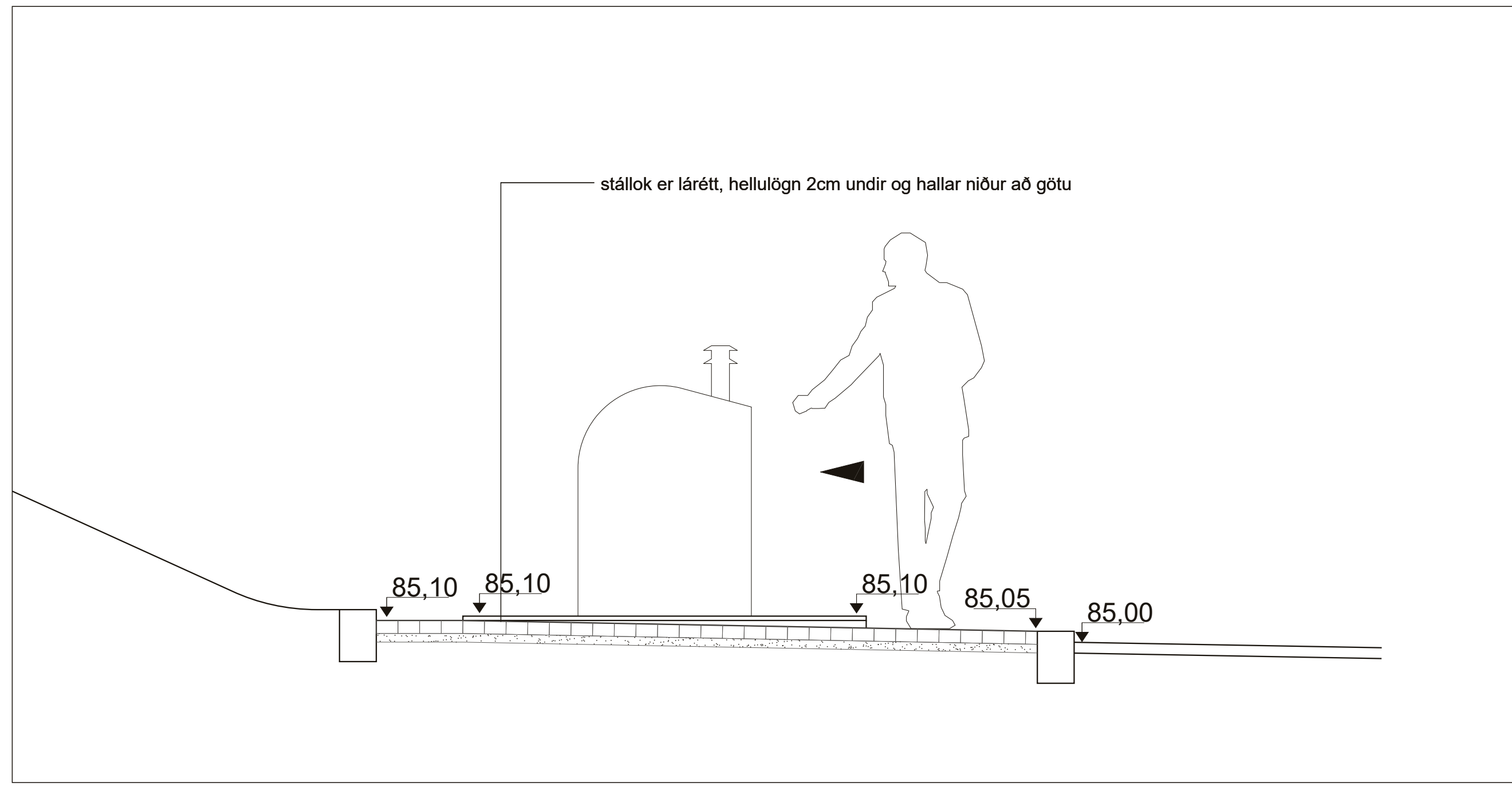
Djúpgámar - snið - mkv. 1:20
