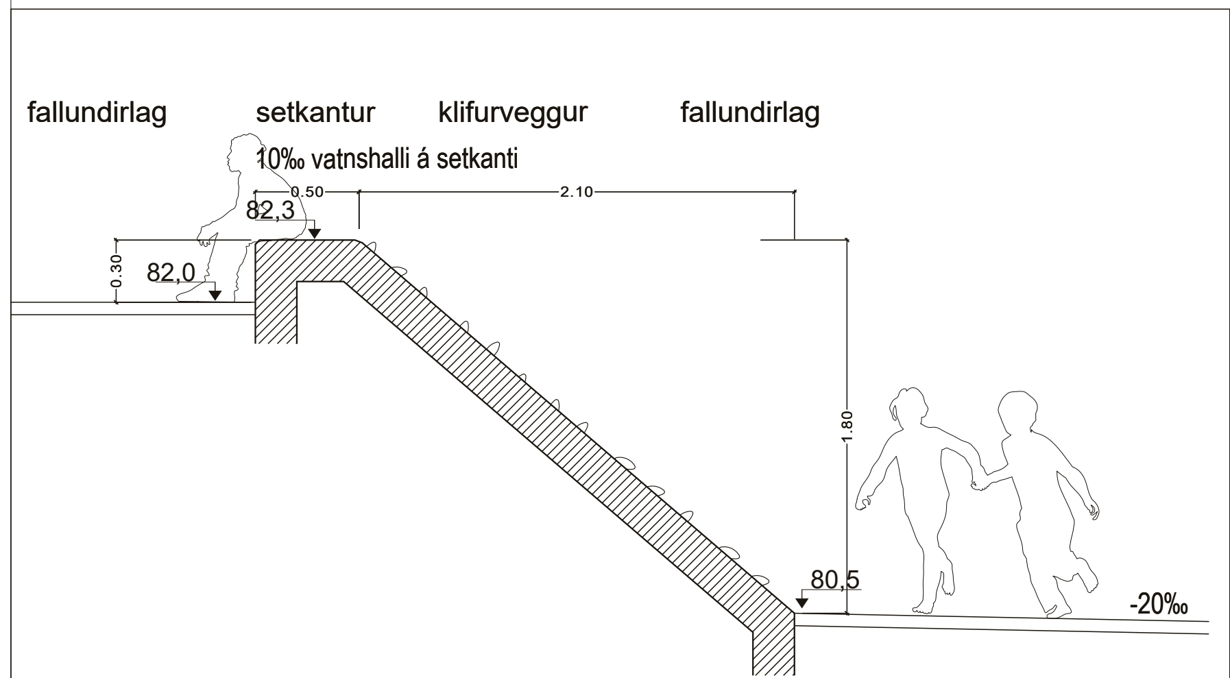
Veggur V-3 - snið b-b - Mkv. 1:25
