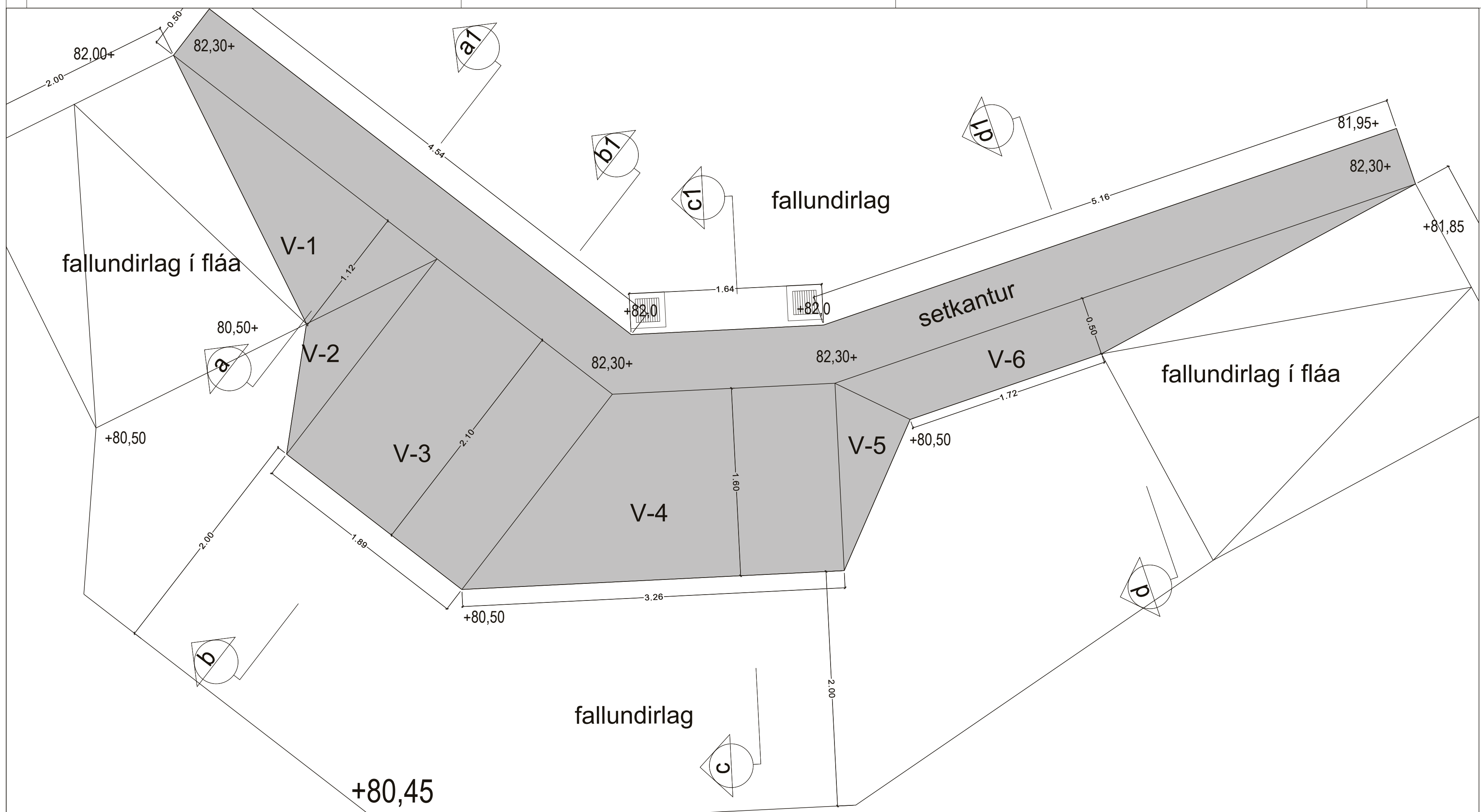
Steyptur klifurveggur - grunnmynd - Mkv. 1:25
