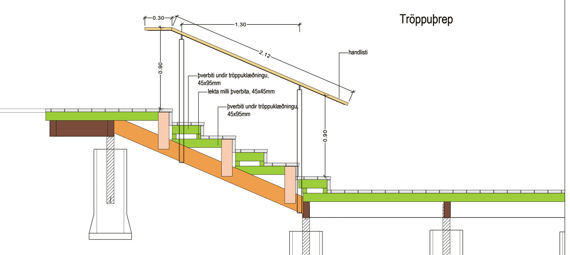
Snið a-a' - Mkv. 1:25
