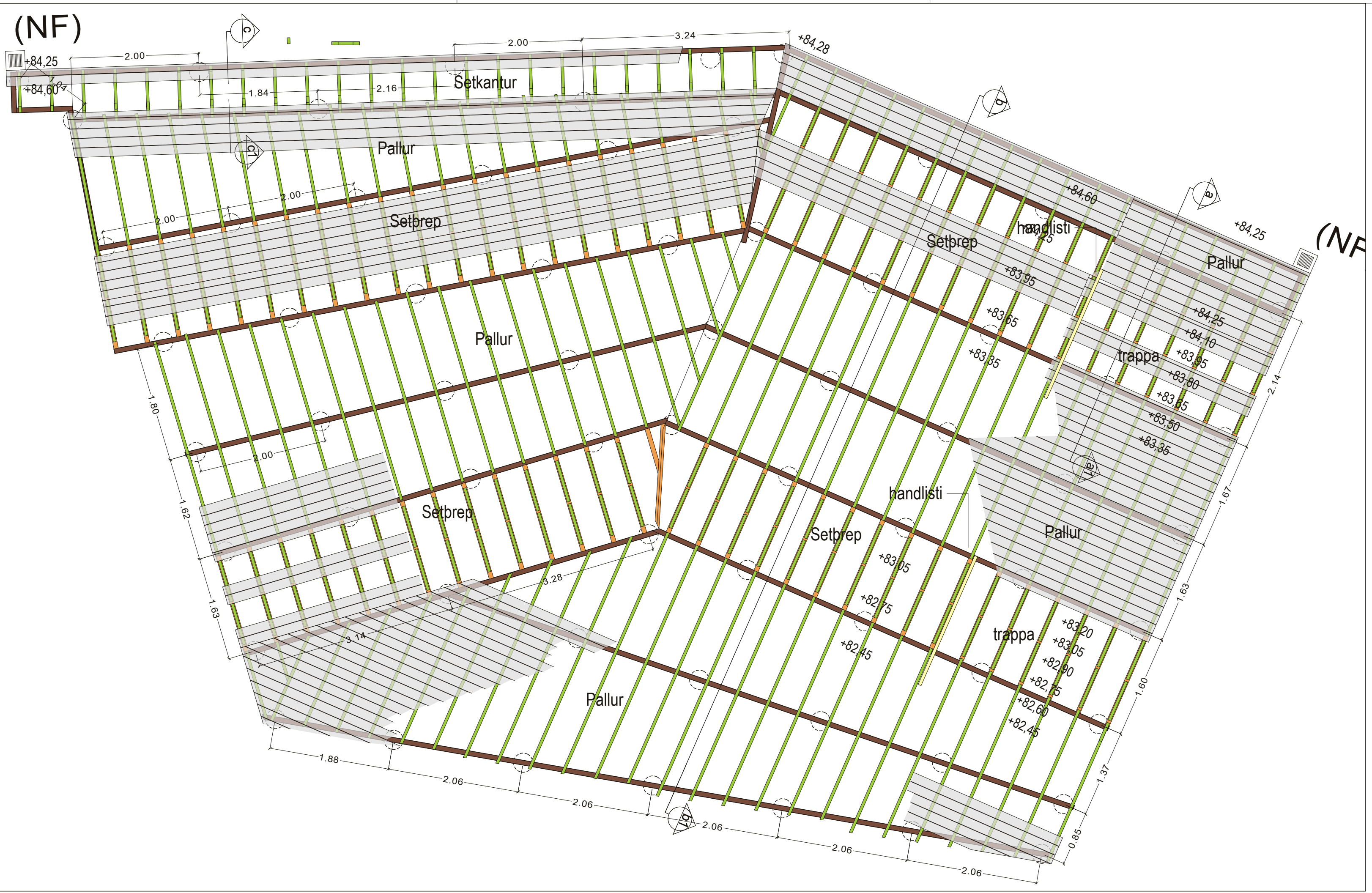
Grunnmynd - Mkv. 1:50
