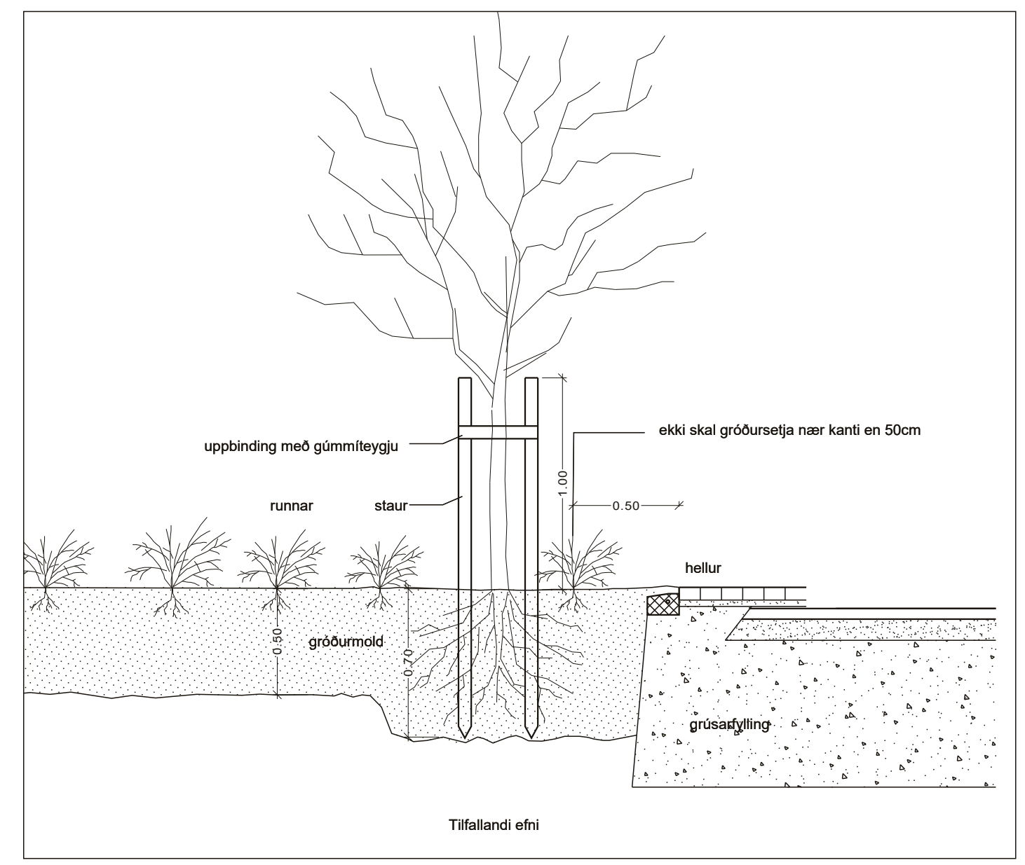
Snið í uppbindingu á trjá - mkv. 1:20
