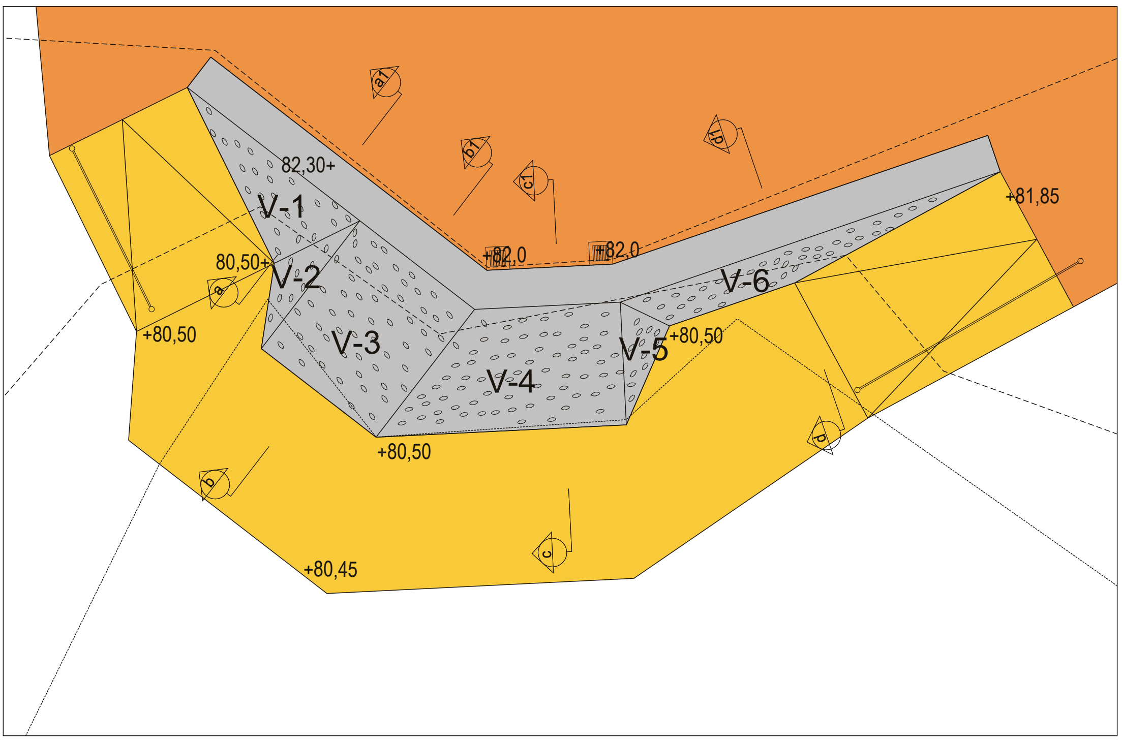
Steyptur klifurveggur - grunnmynd - Mkv. 1:50
