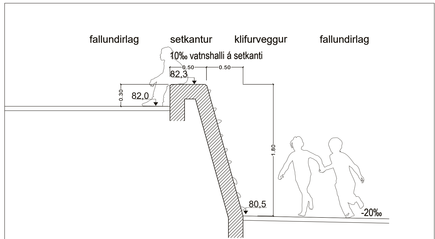
Veggur V-6 - snið d-d - Mkv. 1:25
