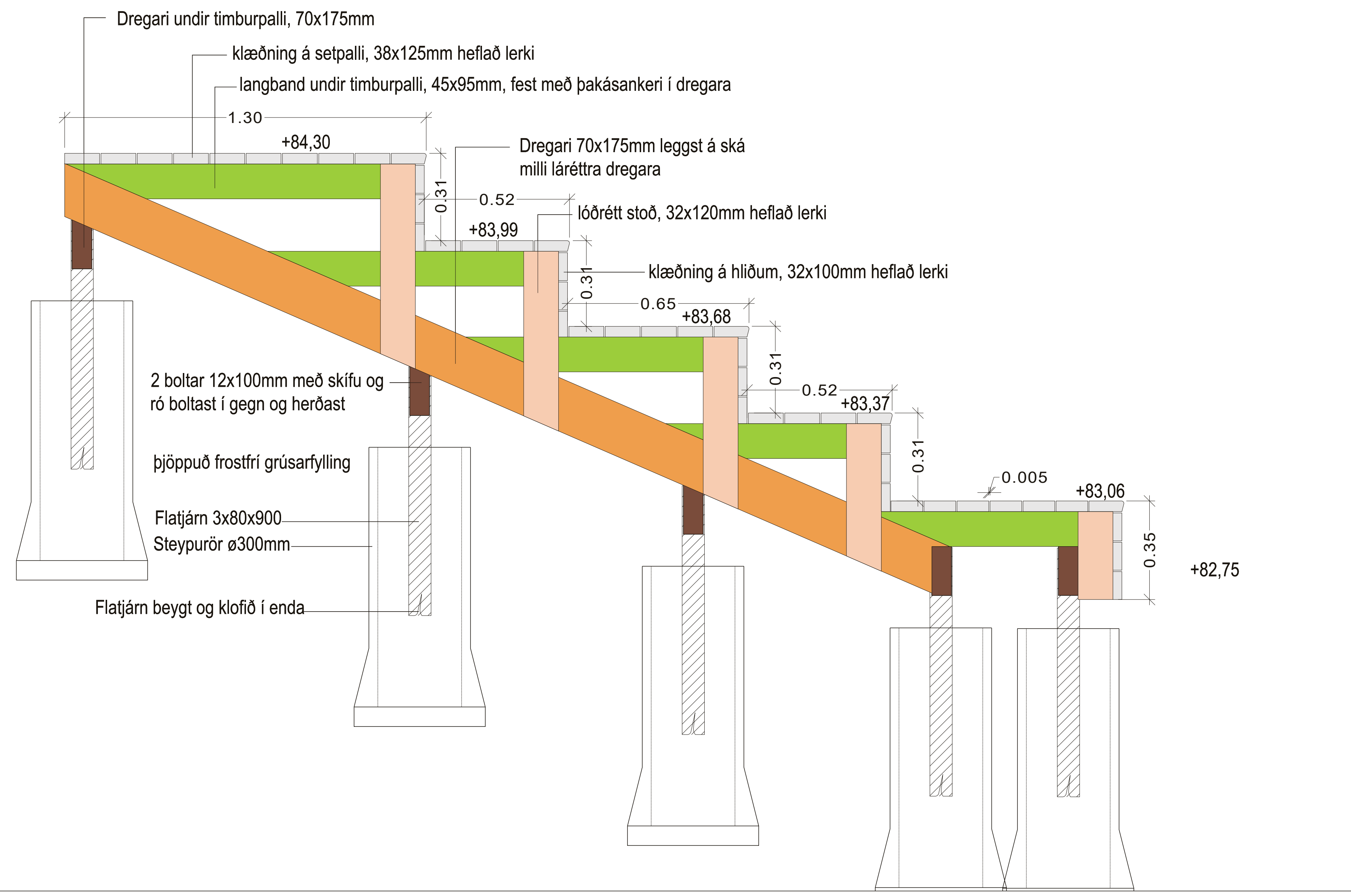
Snið a-a' - Mkv. 1:10
