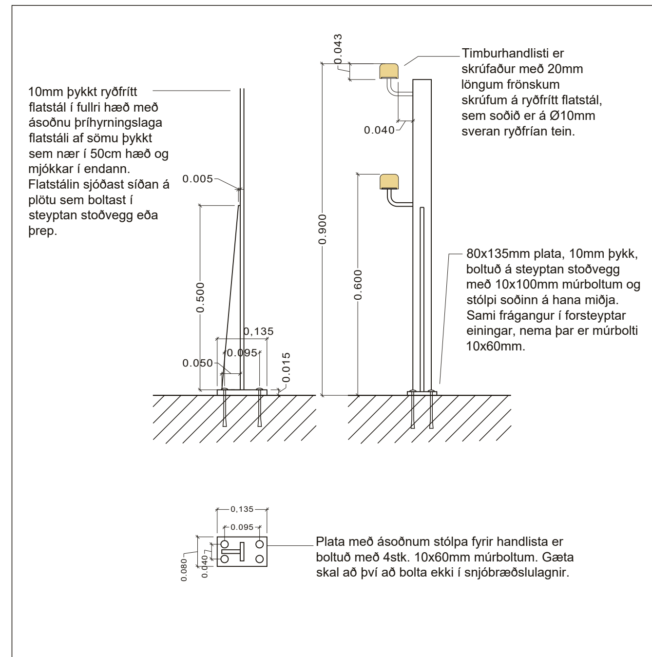
Handlisti og festingar - grunnmynd og snið, mkv. 1:10
