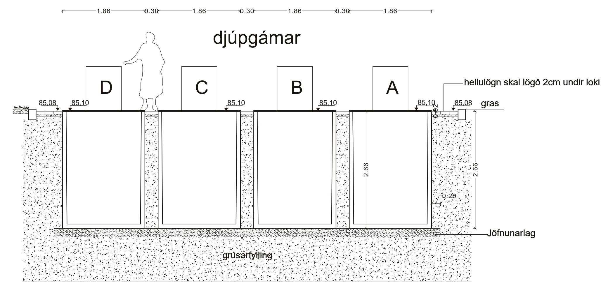
Djúpgámar - grunnmynd og snið - mkv. 1:50
