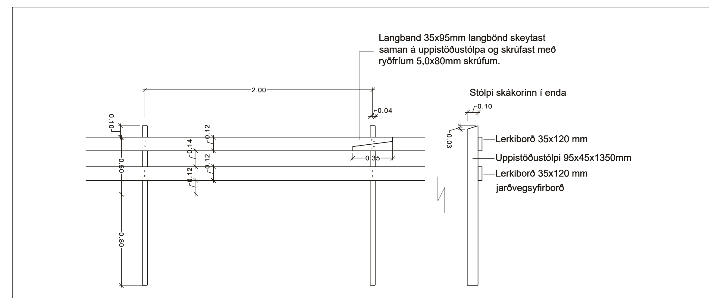
Lágbandagirðin, útlit og snið - mkv. 1:20
