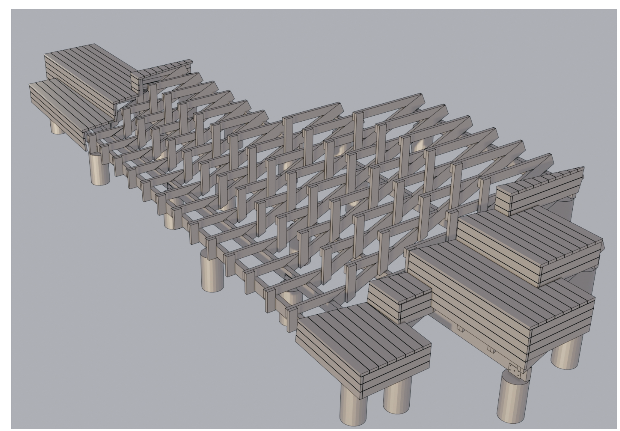
Uppbygging á timburgrind - isometría - ekki í kvarða
