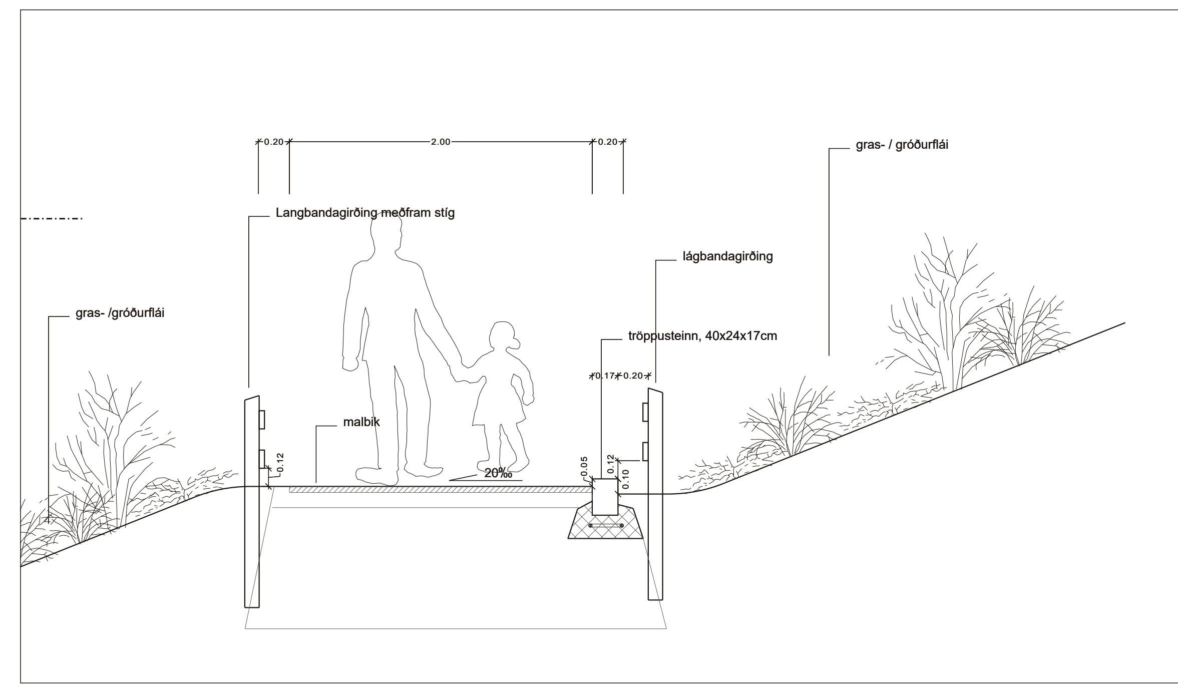
Snið í tröppusteinn neðan við gróðurbeð - mkv. 1:25
