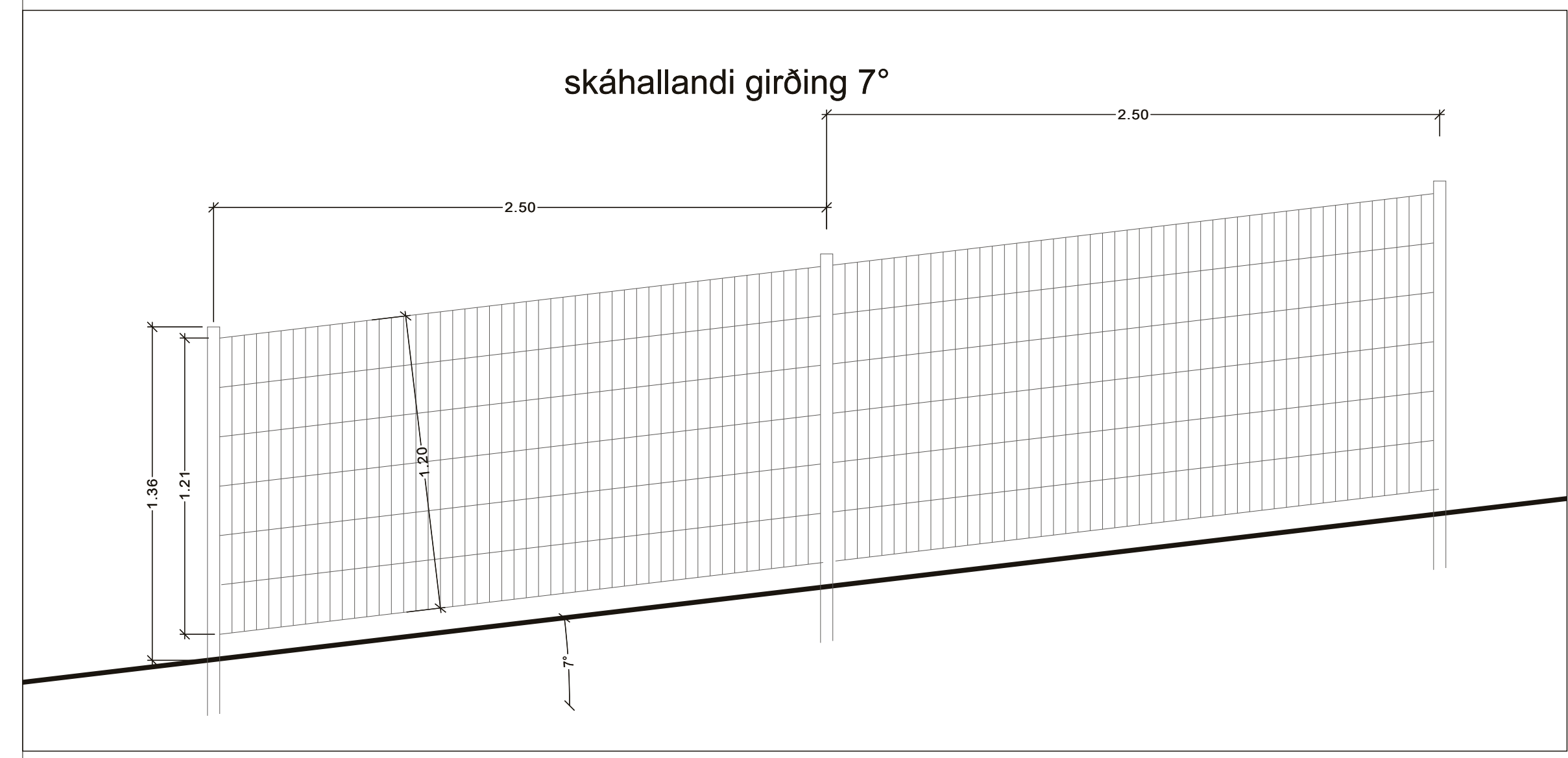
Mkv. 1:20
