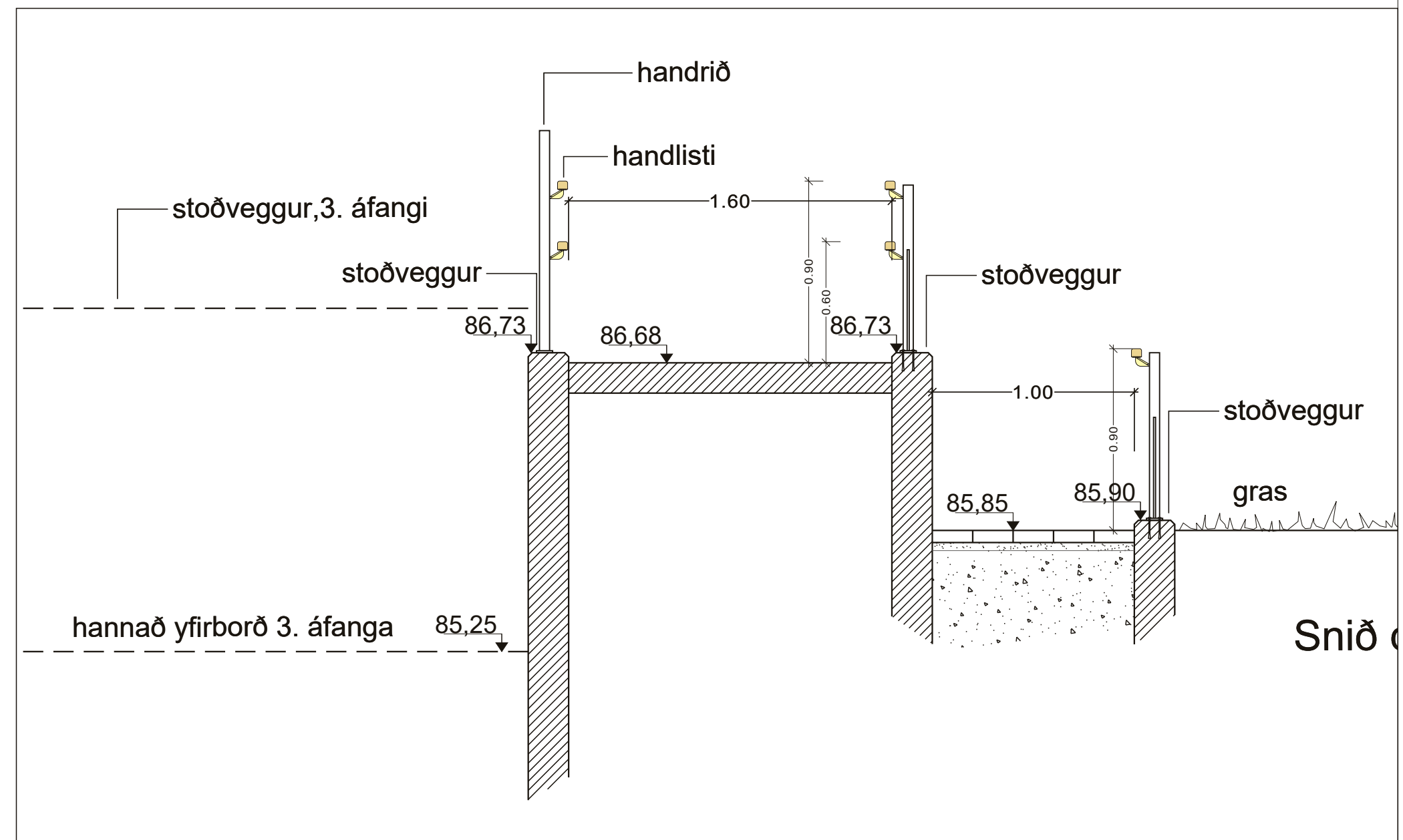
Snið d-d', mkv. 1:25
