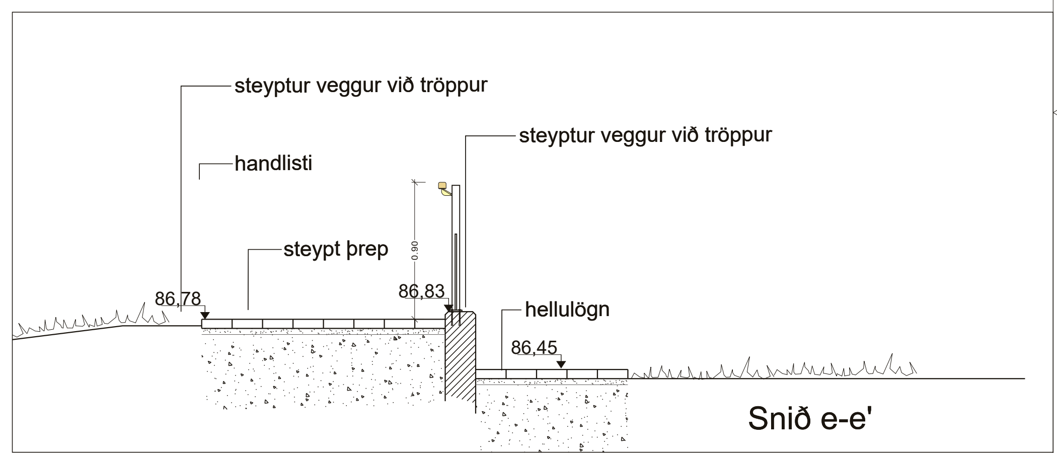
Snið e-e', mkv. 1:25
