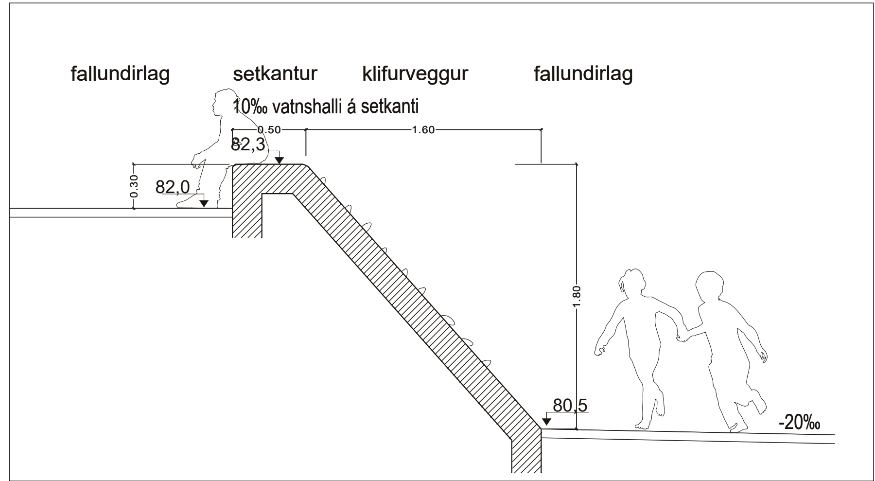
Veggur V-4 - snið c-c - Mkv. 1:25
