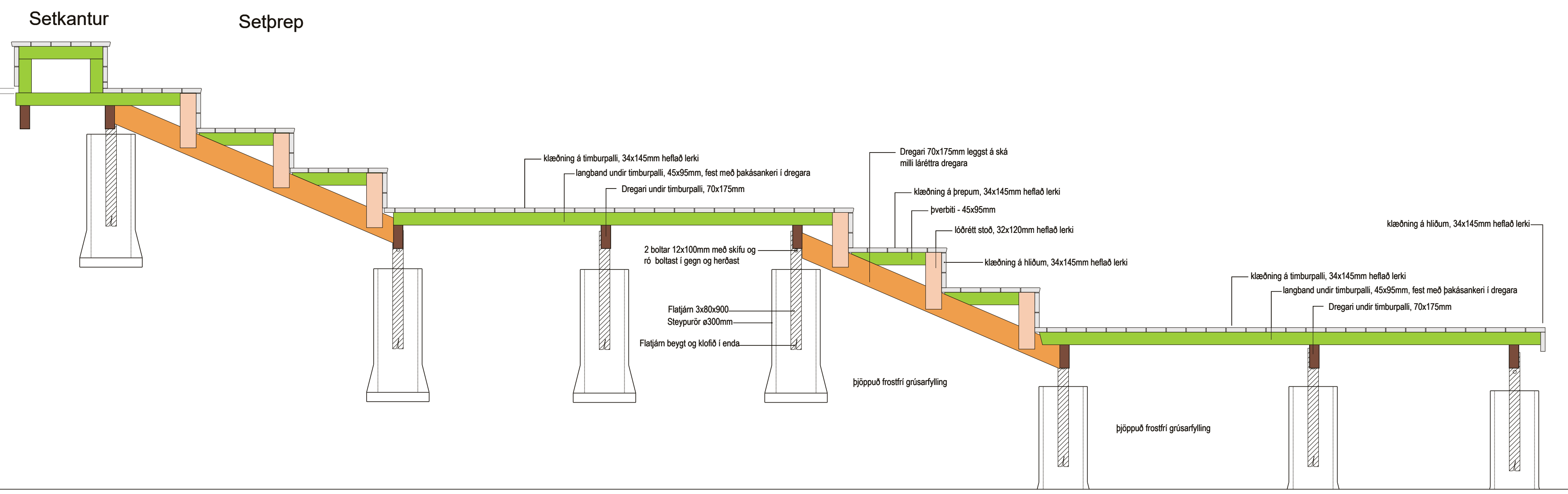
Snið b-b' - Mkv. 1:25
