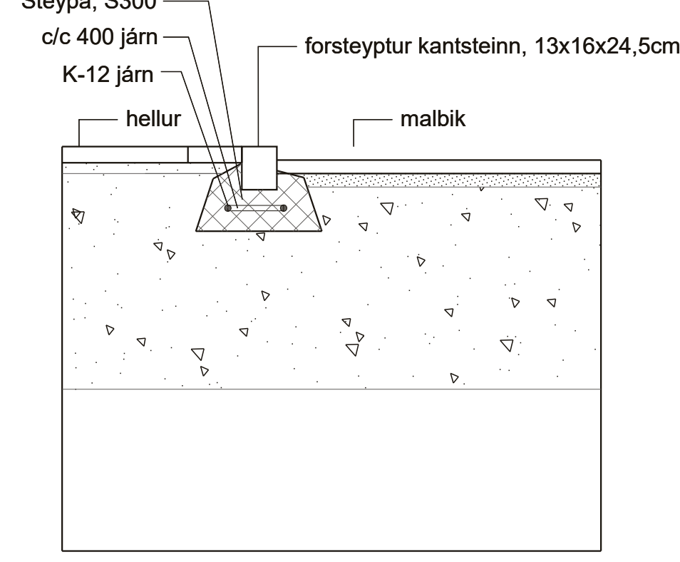
Forsteypur kantsteinn
