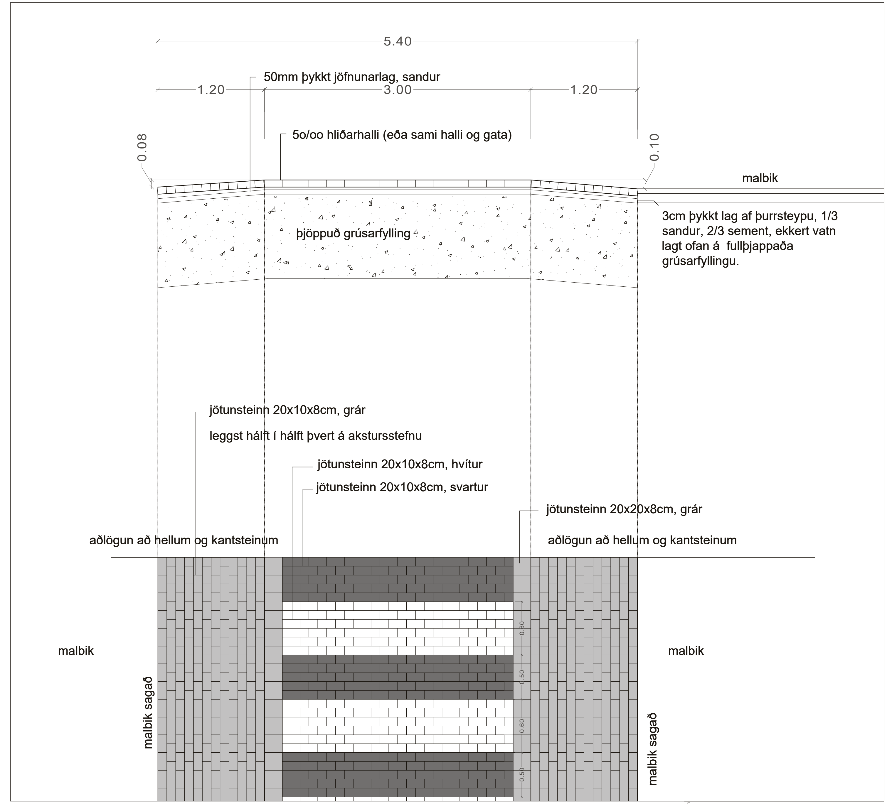
Upphækkuð gangbrauti - grunnmynd og snið - mkv. 1:25
