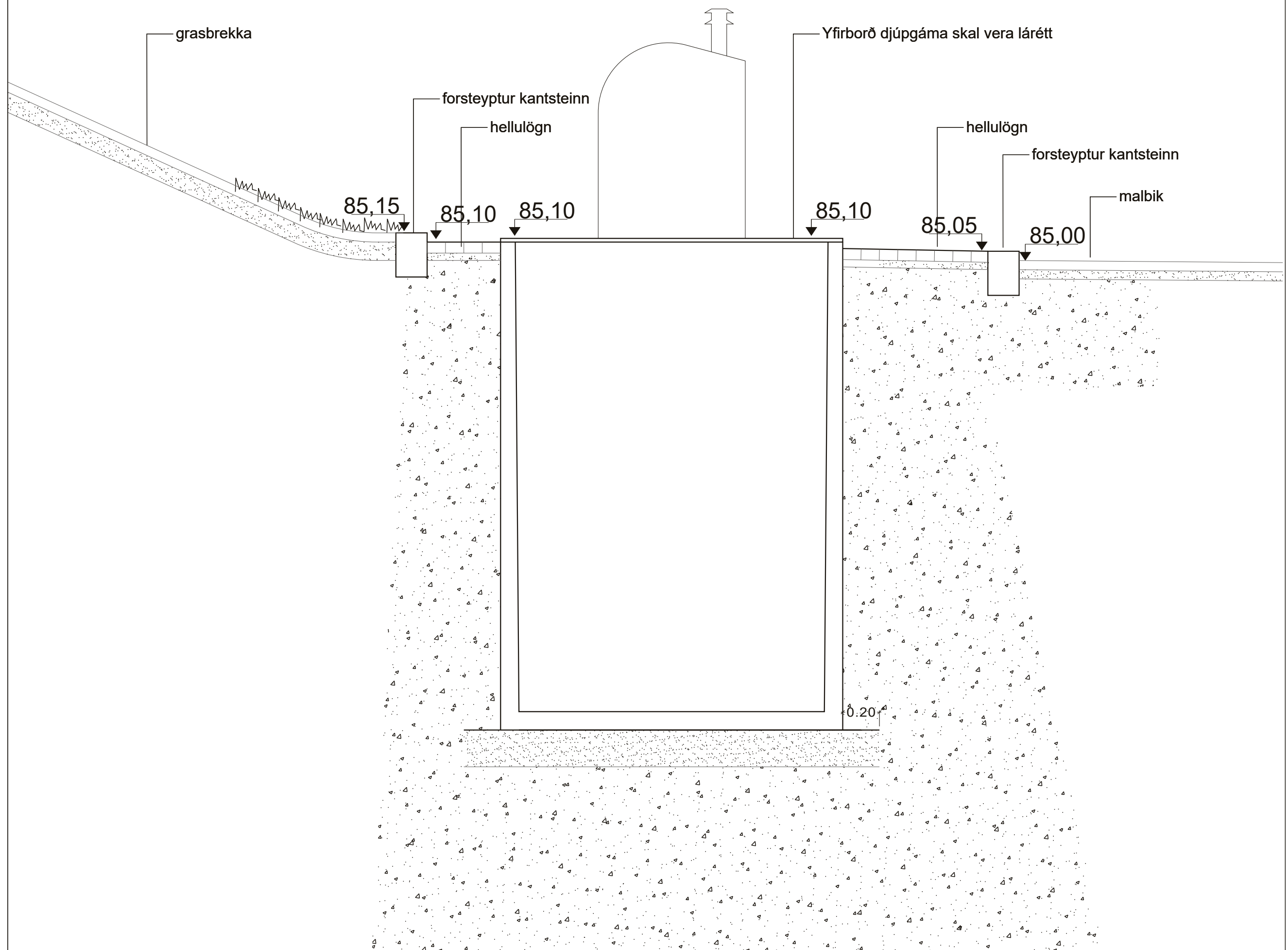
Djúpgámar - grunnmynd og snið - mkv. 1:20
