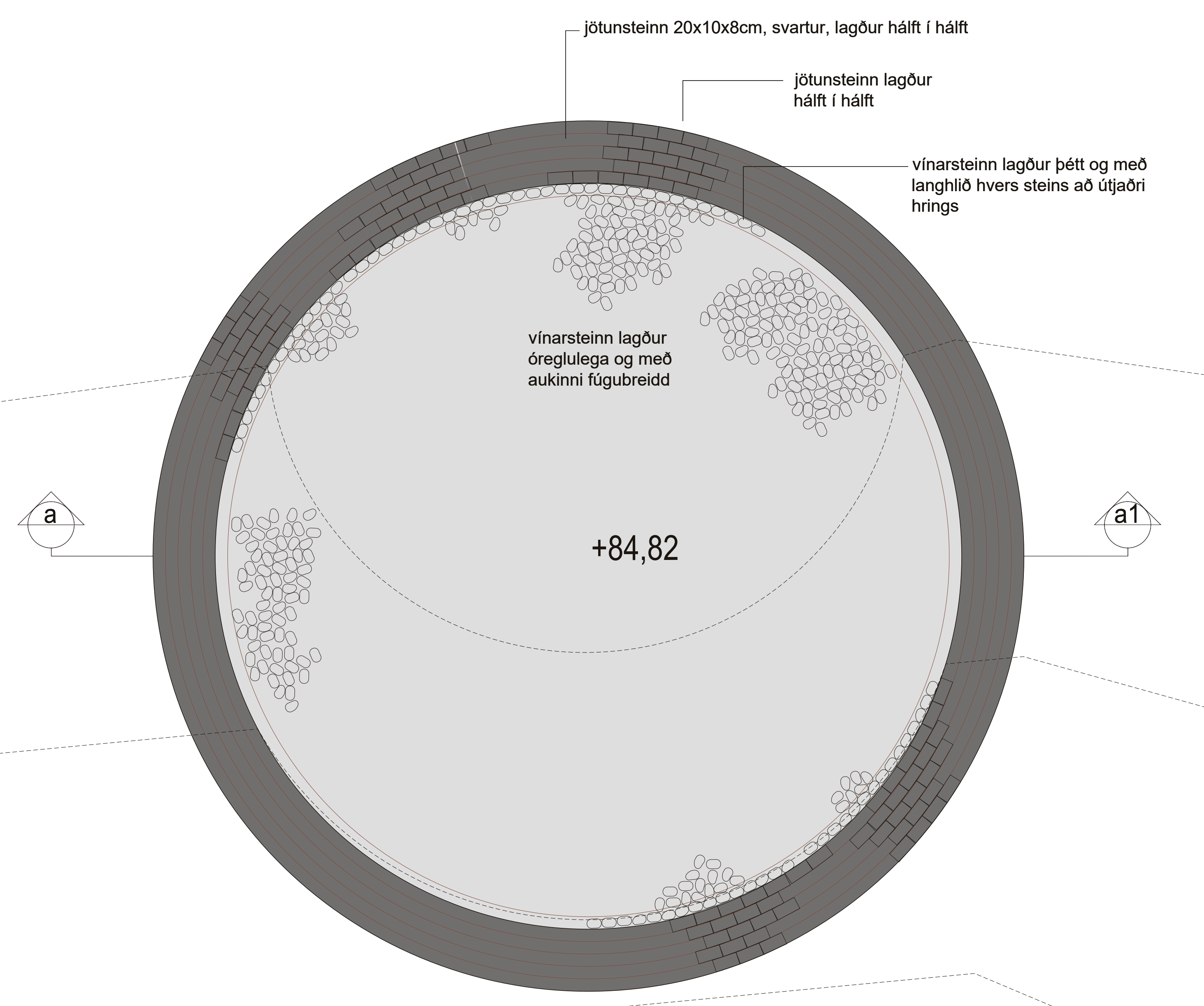
Hellulagt hringtorg við sleppisvæði - grunnmynd og snið - mkv. 1:25
