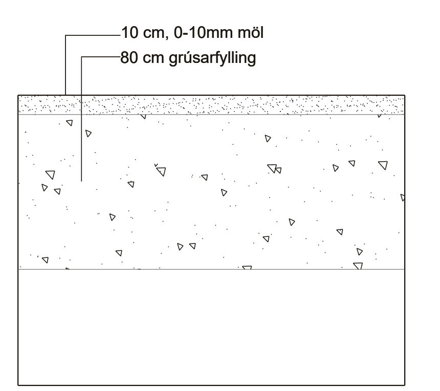
Malarsvæði
