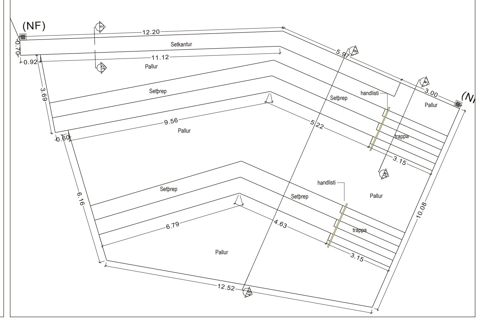
Grunnmynd - þrep og handlisti
